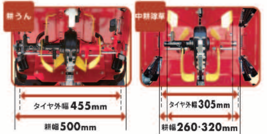
耕幅とトレッド
